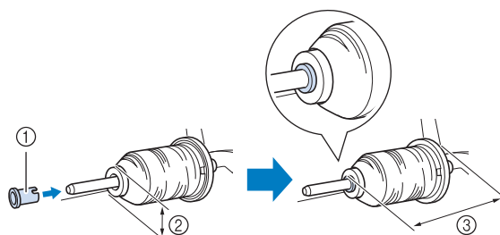
① Couvercle de bobine (spécial) ② 12 mm (1/2 de pouce) ③ 75 mm (3 pouces)
