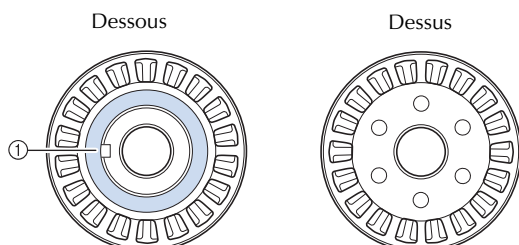
① Aimant
