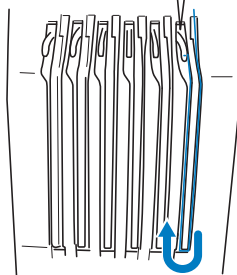
① Levier releveur de fils
