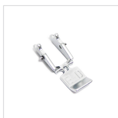
202-155-003 Pied à double entraînement étroit Dual Feed Plus pour fermeture éclair (ED)
